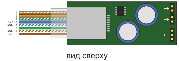
EIA/TIA 568B Канал 2
