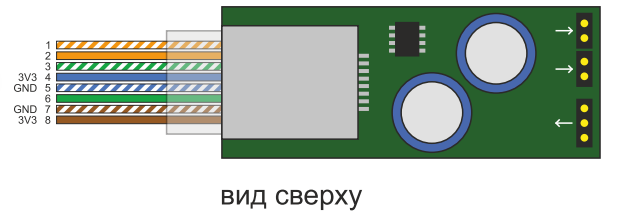
EIA/TIA 568B Канал 4
