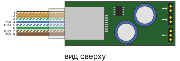
EIA/TIA 568B Канал 3
